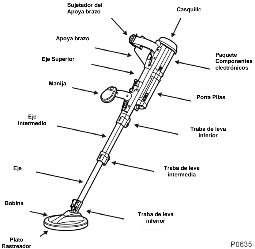
Figura 15: Detector F3
